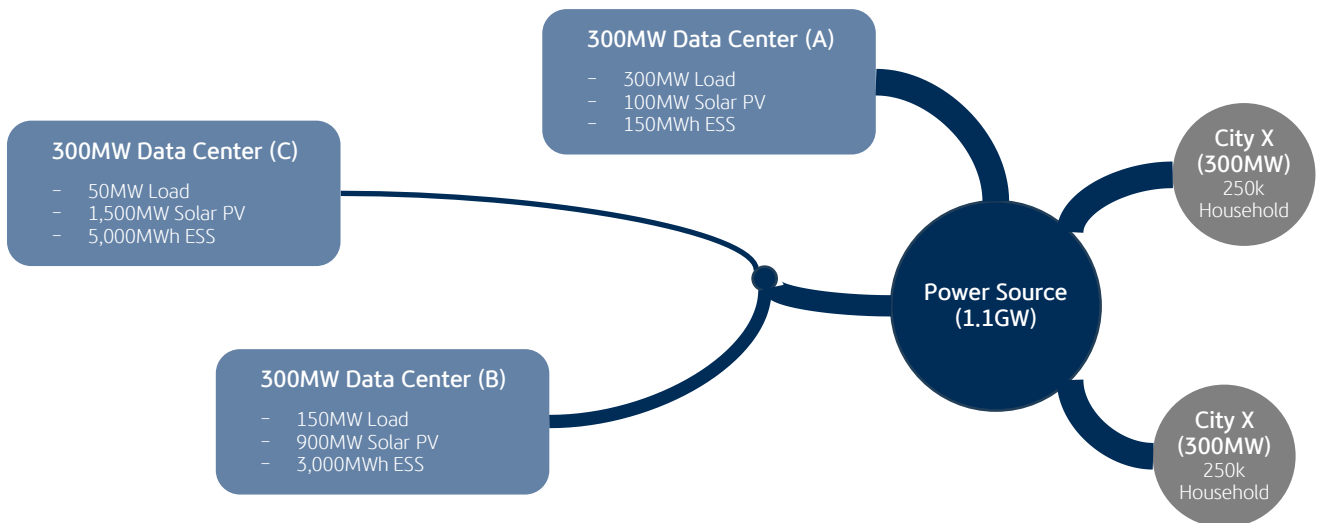
그림 1. 전력망 부족에 따른 태양광/ESS 확대 (A: 2024년, B: 2025년 하반기, C: 2026년)
