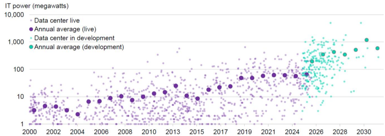
그림 2. 데이터센터 IT Capacity 추이: 심지어 데이터 센터 규모는 확대중
