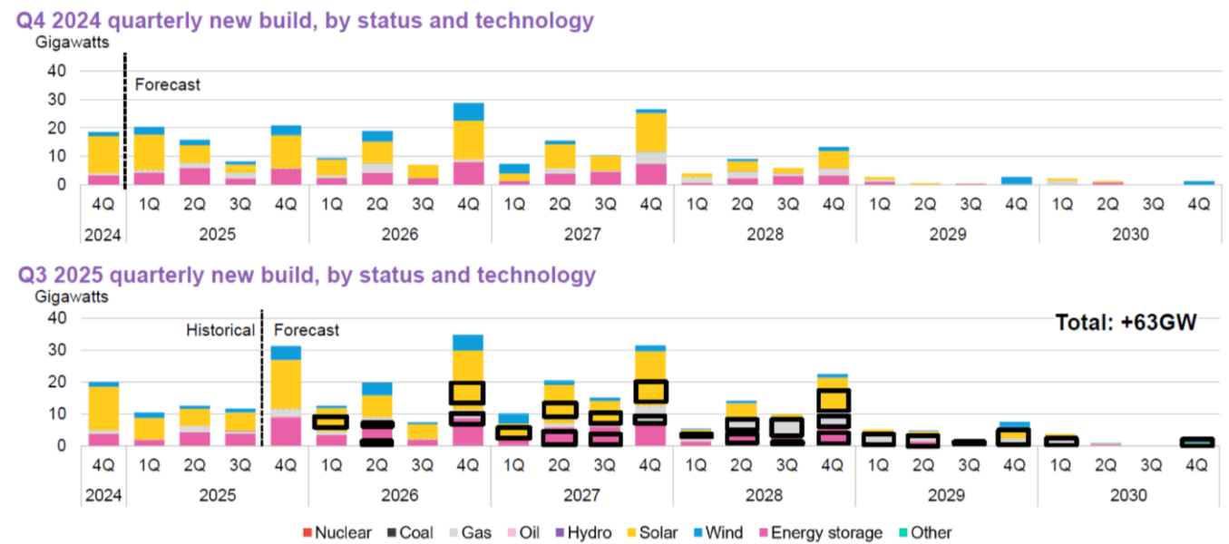
그림 3. 발전원별 신규 설치량 전망 변화: 태양광 크게 추가되는 중
